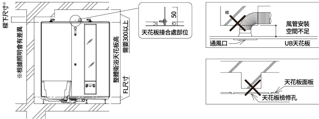
窗戶可開口範圍
