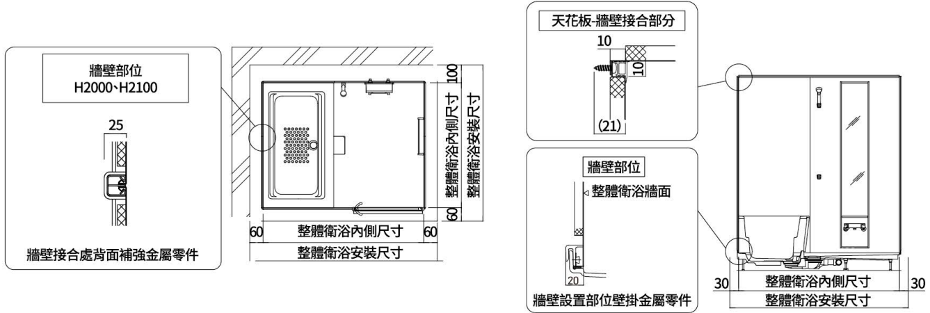
立面結構尺寸
